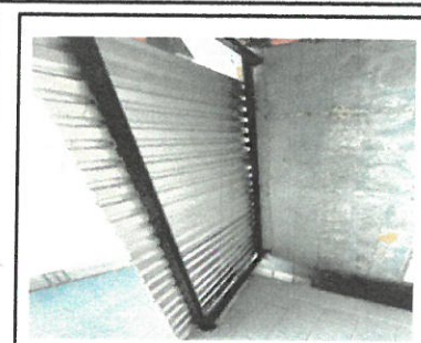
CUBIERTA DE LAMINA, Sustitución de lámina, por lámina troquelada aluzinc calibre 26. ESTRUCTURA DE TECHO, Sustitución de estructura de soporte de madera por metal.
