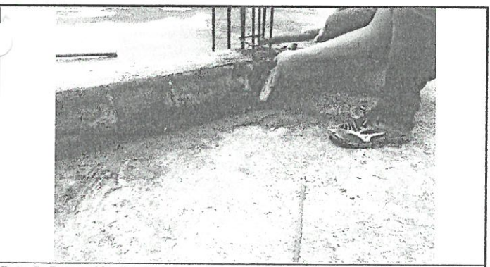
Foto 5: Remoción de sabieta antigua y limpieza de la unión de las paredes.
