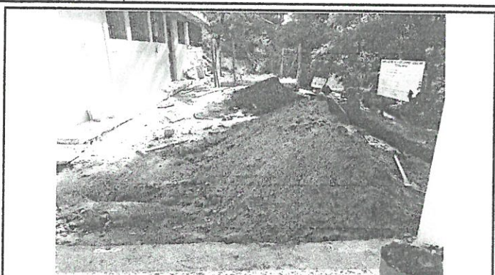
Foto 2: Colocación de pines y compactación de suelo antes de la pavimentación.
