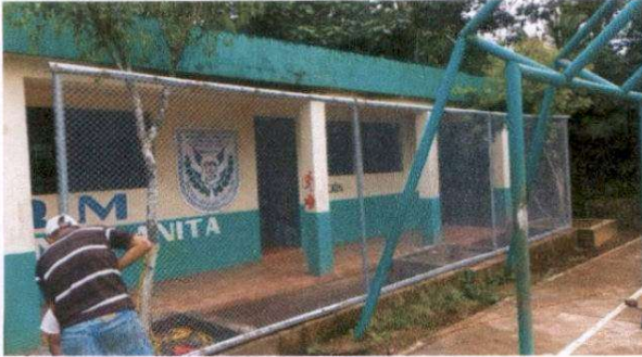
Sustitución de muro perimetral de block con tubo hg y malla galvanizada, soleras intermedias y columnas.
