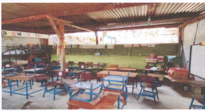
sustitución de estructura de soporte de madera a metal, sustitución de cubierta de lámina por lámina troquelada calibre 26.
