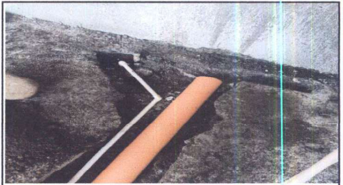
Foto 4: Sustitución de tubería PVC aguas negras
