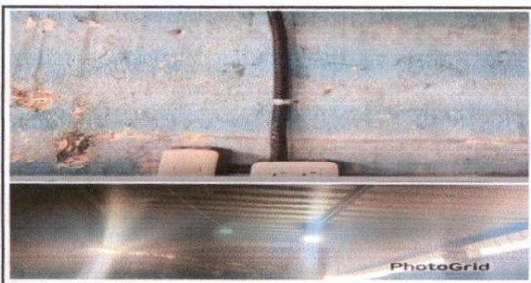
Foto 5: Sustitución de tomacorriente dobles, Focos ahorradores, interruptores simple, ducto electrico, y cableado en cocina
