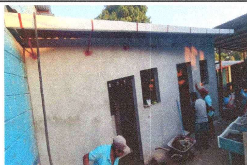
Foto 12: REPARACIÓN DE REPELLO Y CERNIDO DE PAREDES, Se realizó la preparación de la pared para la aplicación de repello y cernido para impermeabilizar.
