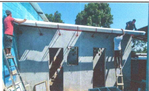
Foto 6: CANALES Y BAJADAS DE AGUA PLUVIAL, Se colocó el canal para el agua pluvial.
