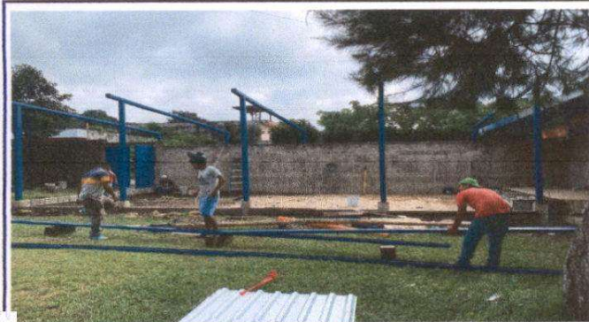
Foto 1: Sustitución de lámina, por lámina troquelada aluzinc calibre 26 de área de patio, sustitucion de piso de torta de concreto y repello de muro perimetral.
