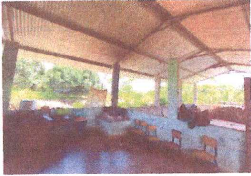
Foto1: Sustitución de malla galvanizada por muro de block en cocina. Mantenimiento a pollerón. Suministro de mueble fijo de concreto revestido de azulejo. Sustitución de piso. Suministro e instalación de balcones.
