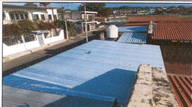
Foto 1: Sustitución de cubierta de lámina por lámina troquelada calibre 24
