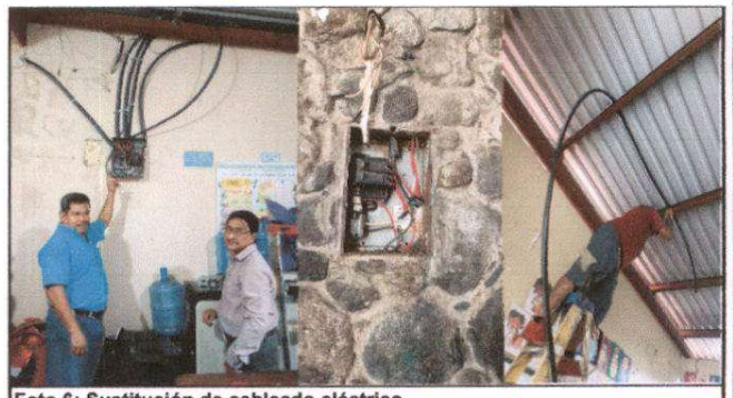
Foto 6: Sustitución de cableado eléctrico (sustitución de flipones, plafoneras, interruptores, tomacorrientes y caja de tablero)
