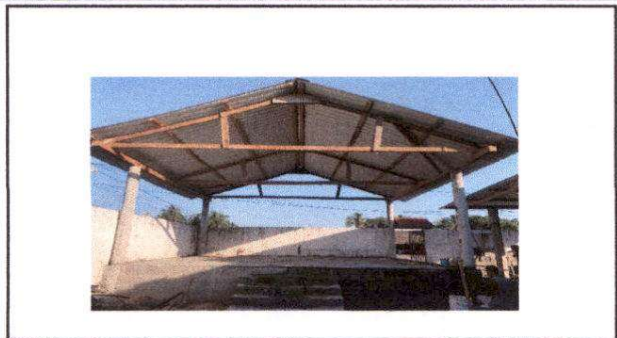
FOTO 1: Suministro de Lamina Troquelada cal. 26, Estructura de Madera y Piso. Escenario
