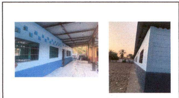
FOTO 3: Aplicación de Pintura en Muros Exteriores
