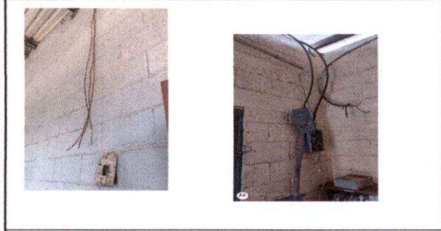
FOTO 5: Suministro de Instalacion de Electricidad de Toda la Escuela
