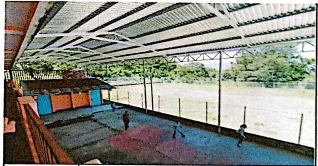
Foto 4: INSTALACIÓN DE TIJERA PARA ESTRUCTURA METALICA
