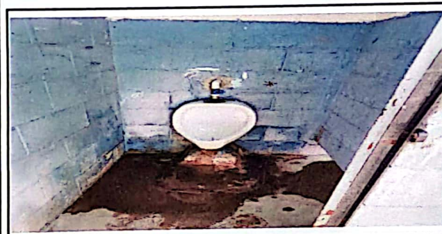
FOTO 3 CAMBIO DE MINGITORIO Y COLOCACION DE PISO CERAMICO Y AZULEJO
