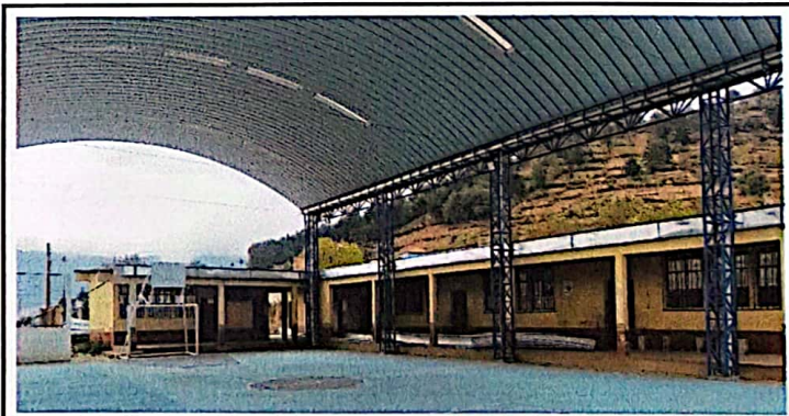
Foto 6: Modulo I Planta Alta, EORM Caserío Palanquix Guachiaquib, pintada de aulas de cuarto y quinto primaria, bodega, interna y externa como también el perímetro o circulación completa de la escuela.
