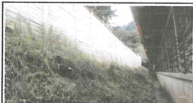
Foto 4: (Muro perimetral y de contención colapsando desde el interior) (Área 2)
