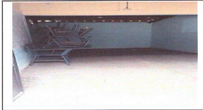
FOTO 12: REDACUACION DE AMBIENTE PARA COCINA, ELABORACION DE ESTUFA DE LEÑA, MUEBLE FIJO MESA DE TRABAJO CON CONCRETO, APERTURA DE VENTANA
