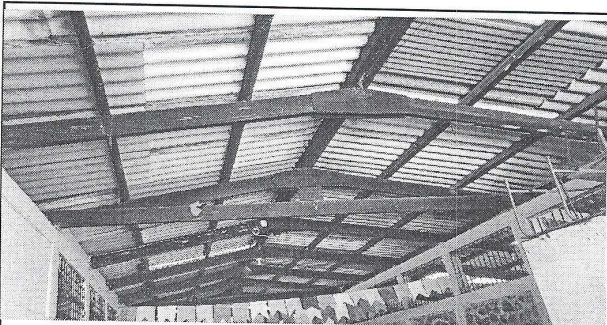
Foto 5: Imagen que muestra el estado actual del techo de duralita y la estructura portante de madera, del módulo de aulas a intervenir.
