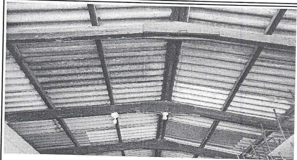
Foto 2: Imagen que muestra el estado actual del techo de duralita y la estructura portante de madera, del módulo de aulas a intervenir.
