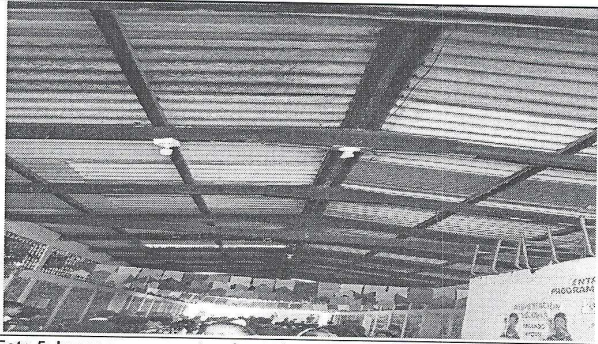
Foto 5: Imagen que muestra el estado actual del techo y la estructura portante de madera, del módulo de aulas a intervenir.
