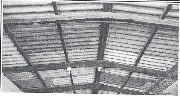
Foto 2: Imagen que muestra el estado actual del techo y la estructura portante de madera, del módulo de aulas a intervenir.
