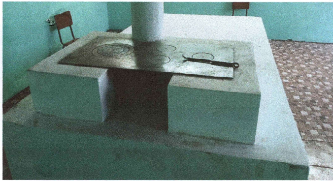
FOTO 1: Finalización de colocación de estufa
