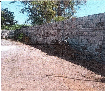
Foto 3: El muro perimetral del lado derecho no cuenta con repello, se prioriza hacer el repello en dicha pared.
