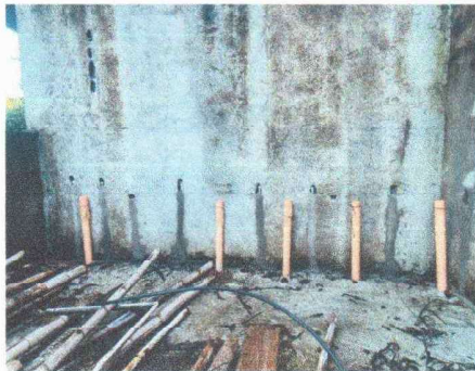
Foto 9: Se observa el área en donde se debe realizar el suministro e instalación de pila de concreto.
