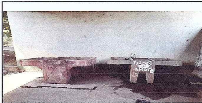
FOTO 5: SE OBSERVA EL DETERIORO DE LA ESTRUCTURA DE CEMENTO EN LAS PILAS.
