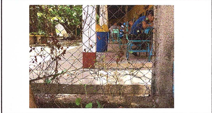
Foto 2: Modulo 1: Reparación de muro perimetral de block con tubo hg y malla galvanizada, soleras intermedias y columnas
