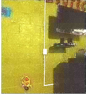
Foto 7: Modulo 2: Sustitución interruptores simples
