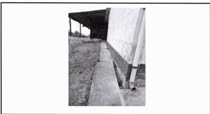
Foto 5: Modulo 1: Sustitución de bajada de agua pluvial de metal por tubo PVC 3"
