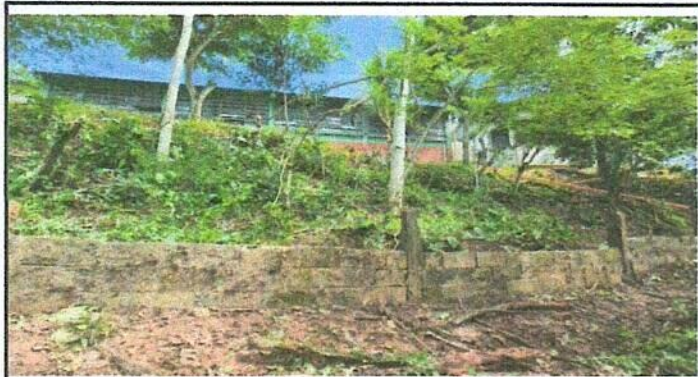
Foto 1: Muro de contención, levantado de muro con blok de arena, soleras intermedias y columnas
