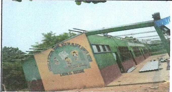
Foto 2: ESTRUCTURA DE TECHO. SUSTITUCION DE SOPORTE DE MADERA, POR METAL
