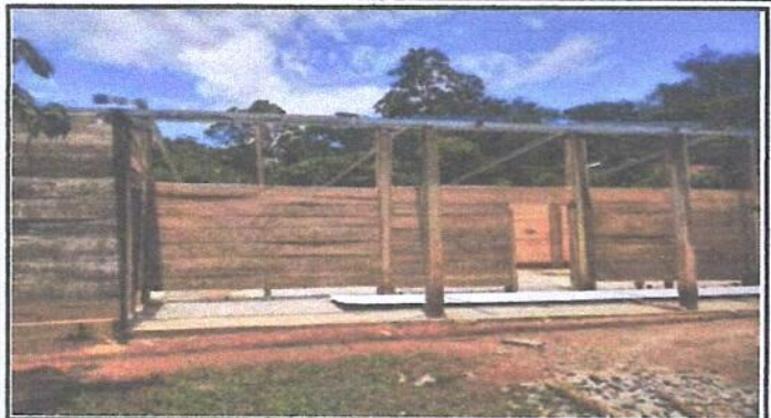
Foto 2: Sustitución de estructura de soporte de madera, por metal del centro educativo
