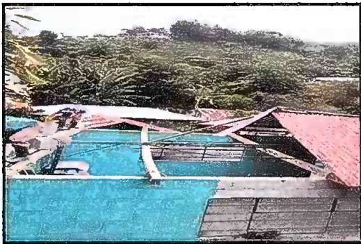
Foto 5: MÓDULO 1 Sustitución de elementos de fijación (tornillos)
