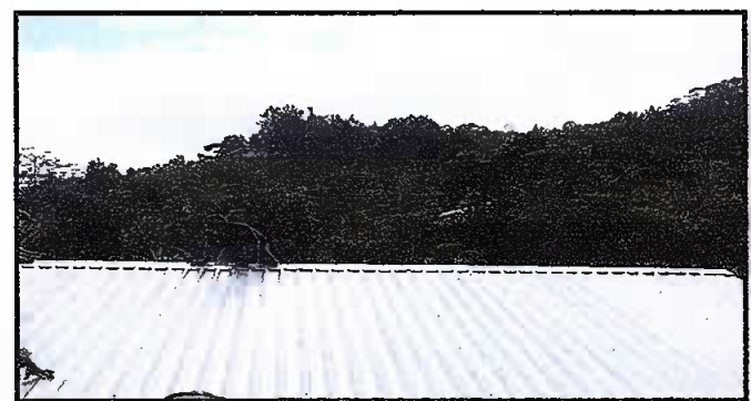
Foto 4: MÓDULO 1 Sustitución de capote de lámina para lámina troquelada
