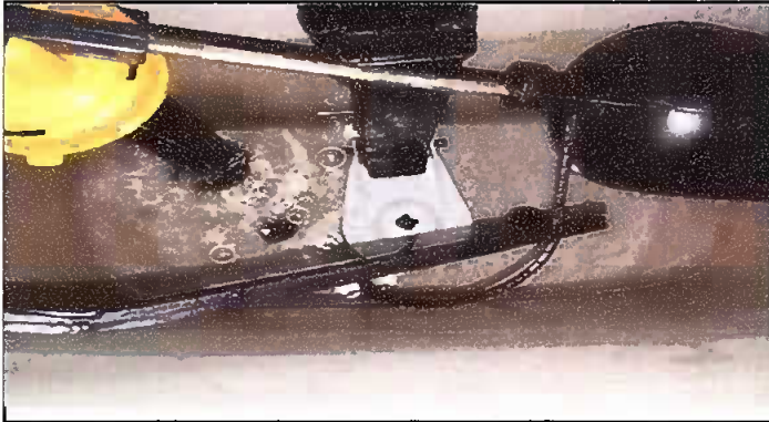
Foto13: SUSTITUCIÓN DE ACCESORIOS DE INODORO(CONTRA LEVE, TUBO DE ABASTO Y TANQUE). MODULO IV.
