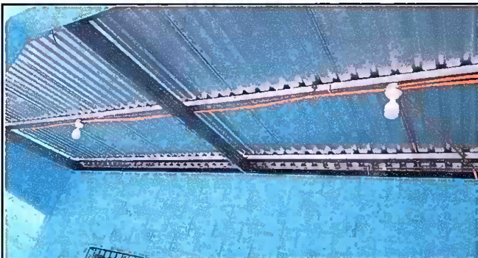
Foto1: Modulo 1. Sustitución de lamina de duralita por lamina troquelada, costanera y canaletas fluviales.
