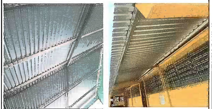
Foto 2: Estructura de soporte de metal galvanizado del módulo uno.
