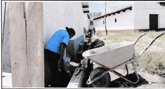
Foto 3: Reparación de muro perimetral de bloques con tubo de hierro y malla galvanizada, soleras intermedias y columnas.
