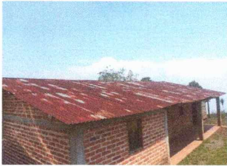
Foto1: Modulo 1: Sustitución de lámina, por lámina troquelada aluzinc calibre 26
