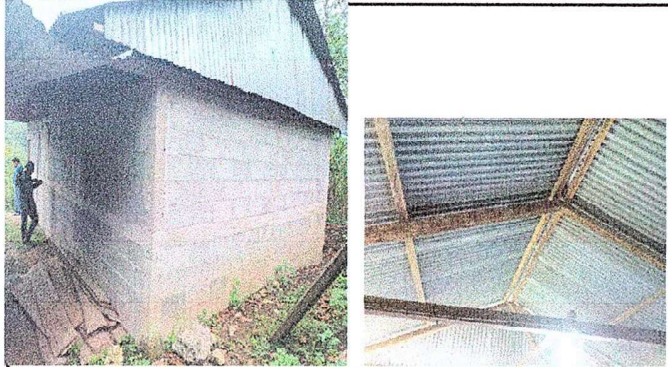
MODULO 1. Foto No. 1y 2 Sustitucion de lamina, por lamina troqueladaa luzinc calibre 26 Sustitucion de capote de lamina para lamina troquelada
