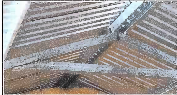
Foto 3: Sustrucción de estructura de soporte de madera por metral
