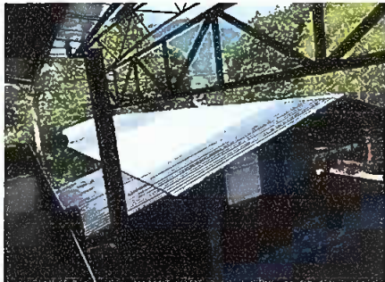
Foto1: Vista de Techo de modulo terminado
