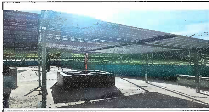
Foto 5: Sustitución de lámina, por lámina troquelada aluzinc calibre 26 y Sustitución de estructura de soporte de madera, por metal.
