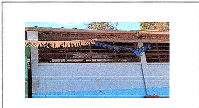
Modulo 2 Suministro e instalación de canal de metal e instalación de bajada de agua pluvial
