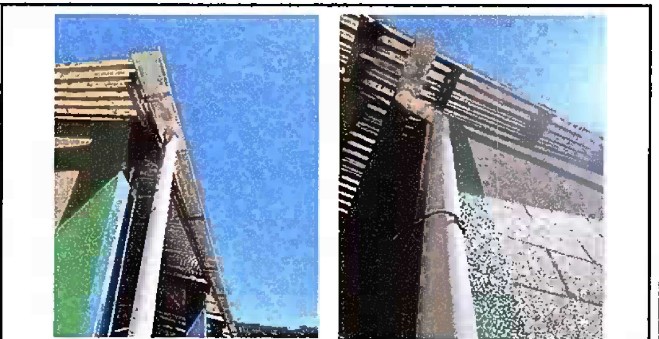
Foto 6: Modulo 1: Sustitución de bajada de agua pluvial de metal por tubo PVC 3"
