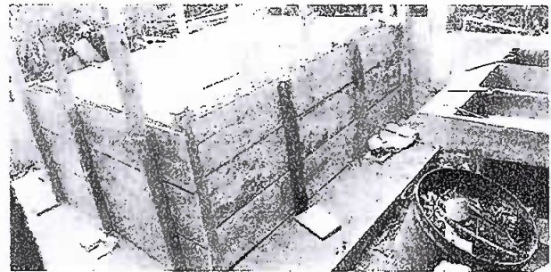
Foto 4: Modulo 1. Esta es la construccion de la pila de de 4 lavaderos, aquí es donde estan formateando.
