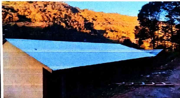
Foto1: Módulo 1. Sustitución de lámina duralita, por lámina troquelada aluzinc calibre 24.
