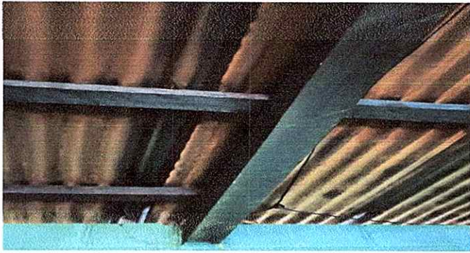
Módulo 1: Sustitución de lámina por lámina troquelada y sustitución de estructura portante de madera por metal.
