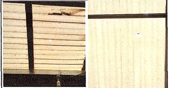
Módulo 2 Instalación de lámina troquelada aluzinc calibre 26 de 12 pies
