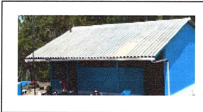
Foto 1: Sustitución de lámina a lámina troquelada aluzinc, calibre 26
