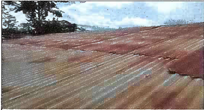
Foto 3: Módulo 4 Sustitución de láminas, por láminas troquelada aluzinc calibre 26
