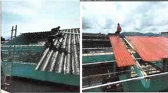
Fotografía 1. MODULO 1: Sustitucion de lámina (duralita) capote y elementos de fijación (tornillos) por lámina troquelada.
