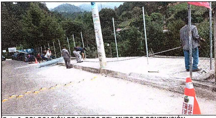
Foto 5: COLOCACIÓN DE HIERRO DEL MURO DE CONTENCIÓN
