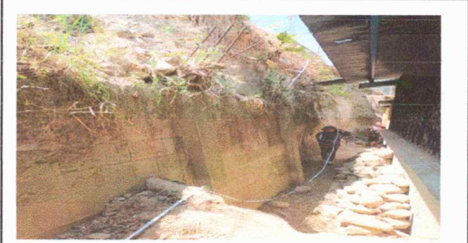
Foto1: REPARACION DE MURO DE CONTENCIÓN
